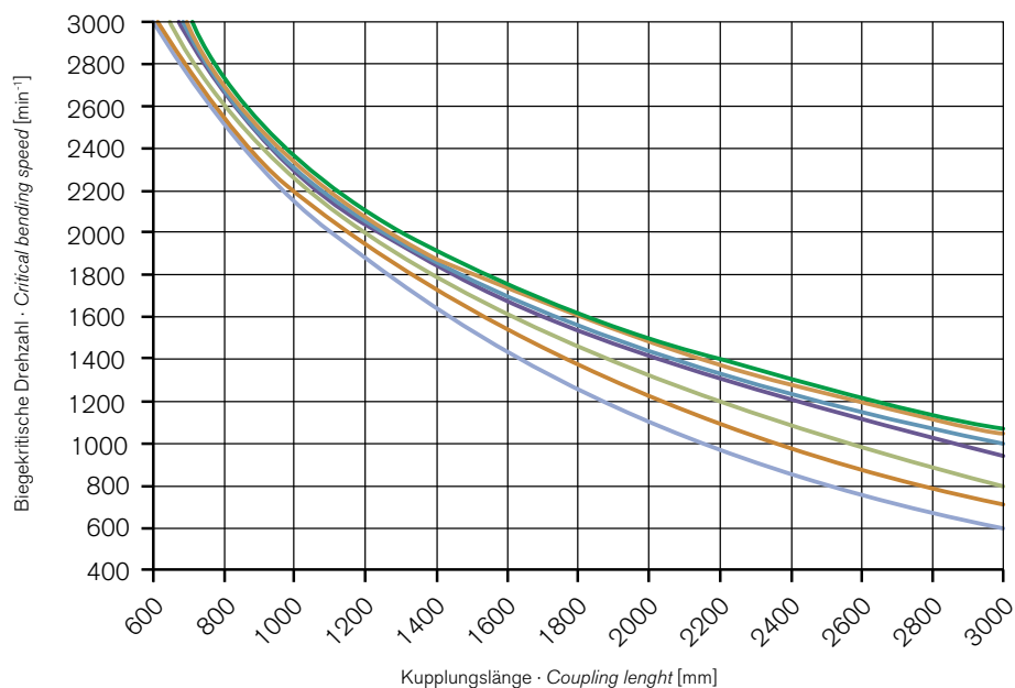
GWZ 5106
